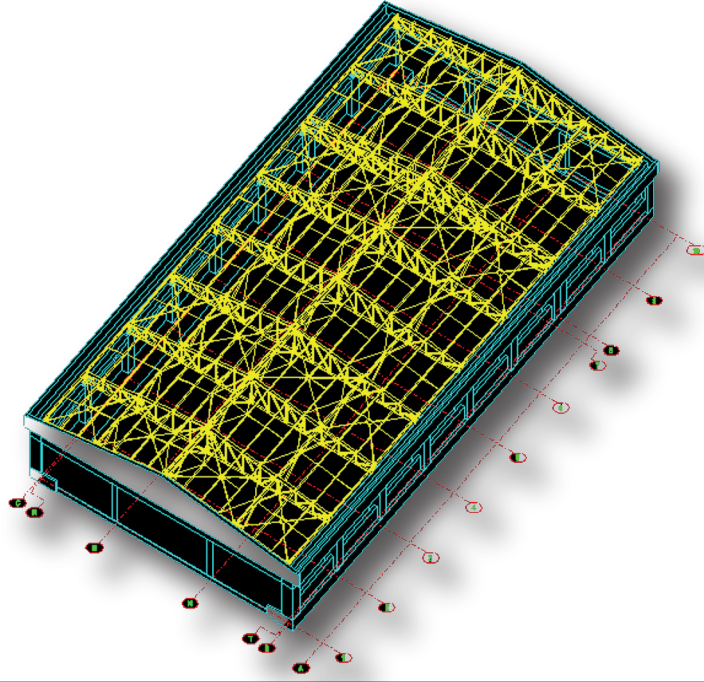
Kızılağaç HEPP Powerhouse Roof
